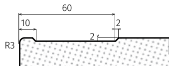
standardní frézování
